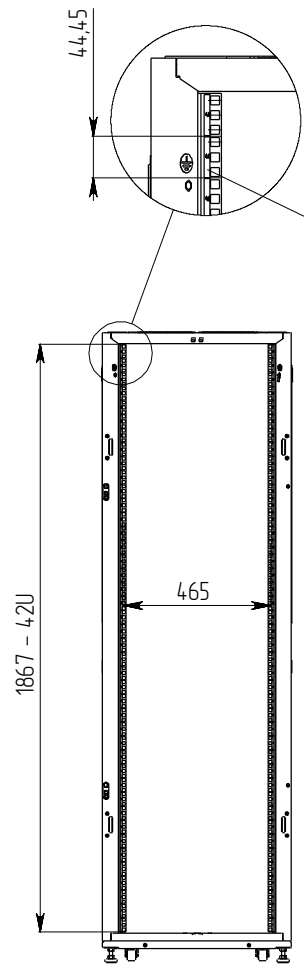
Вид спереди Дверь условно не показана
