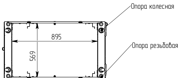
Вид снизу
