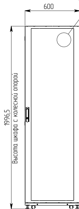
Вид спереди
