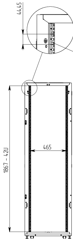
Вид спереди
